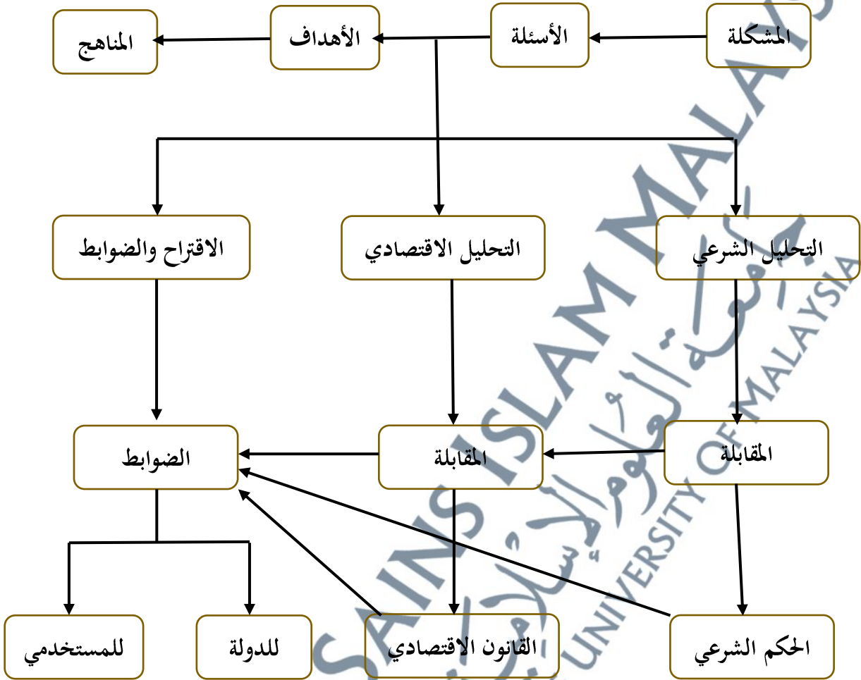
شكل ٢ : هيكل البحث
